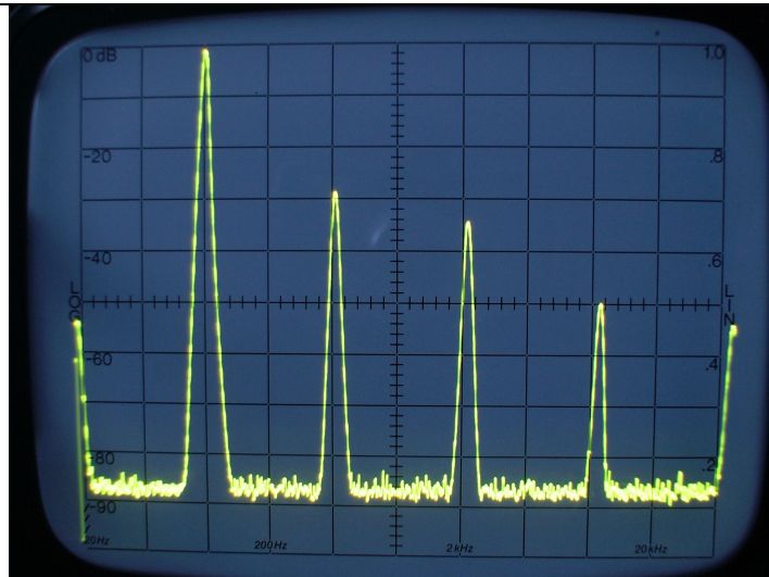
DHT 10 KHz – 5 KHz / Div
