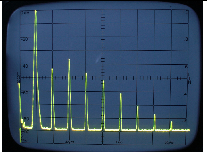
DHT 1 KHz – 1KHz / Div
