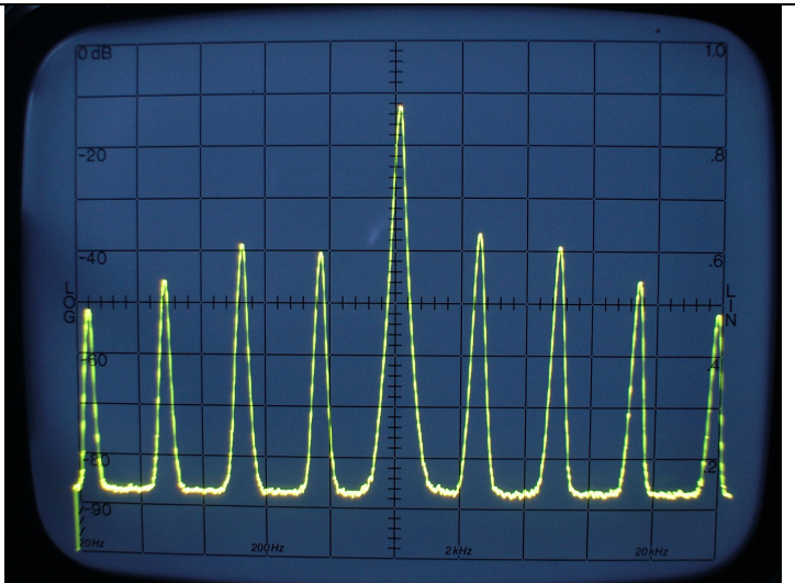
DIM 60 Hz + 7 KHz – Fc 7 KHz – 50 Hz / Div
