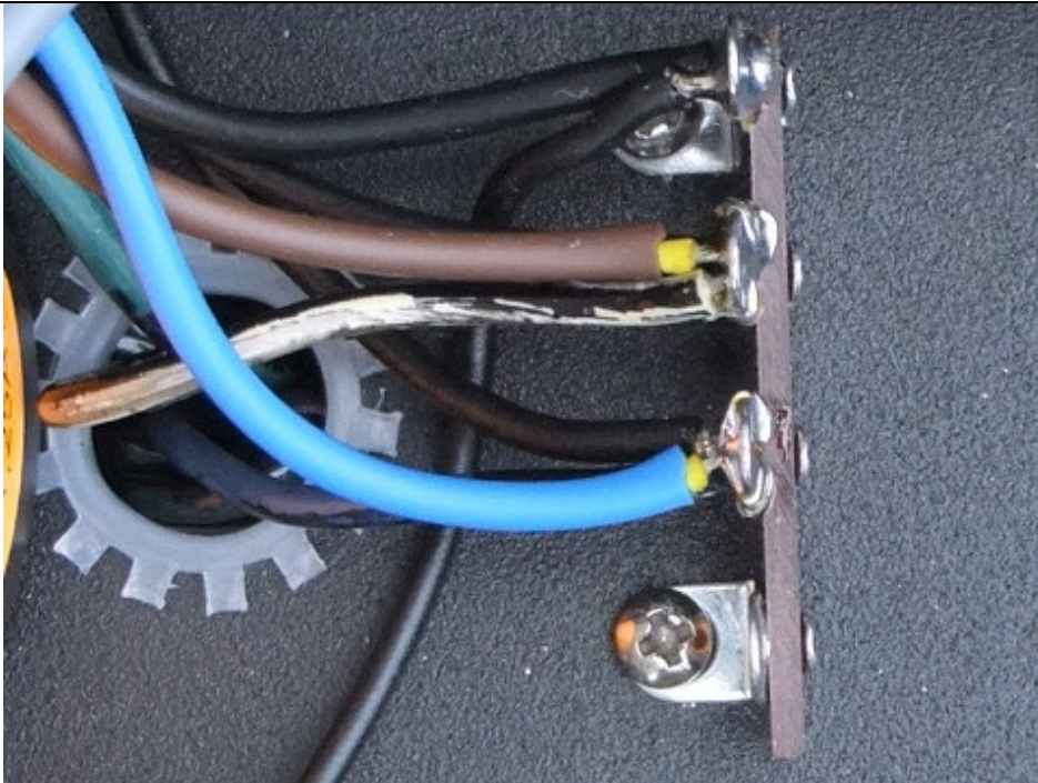
Barette relais 1 : raccordement des primaires
