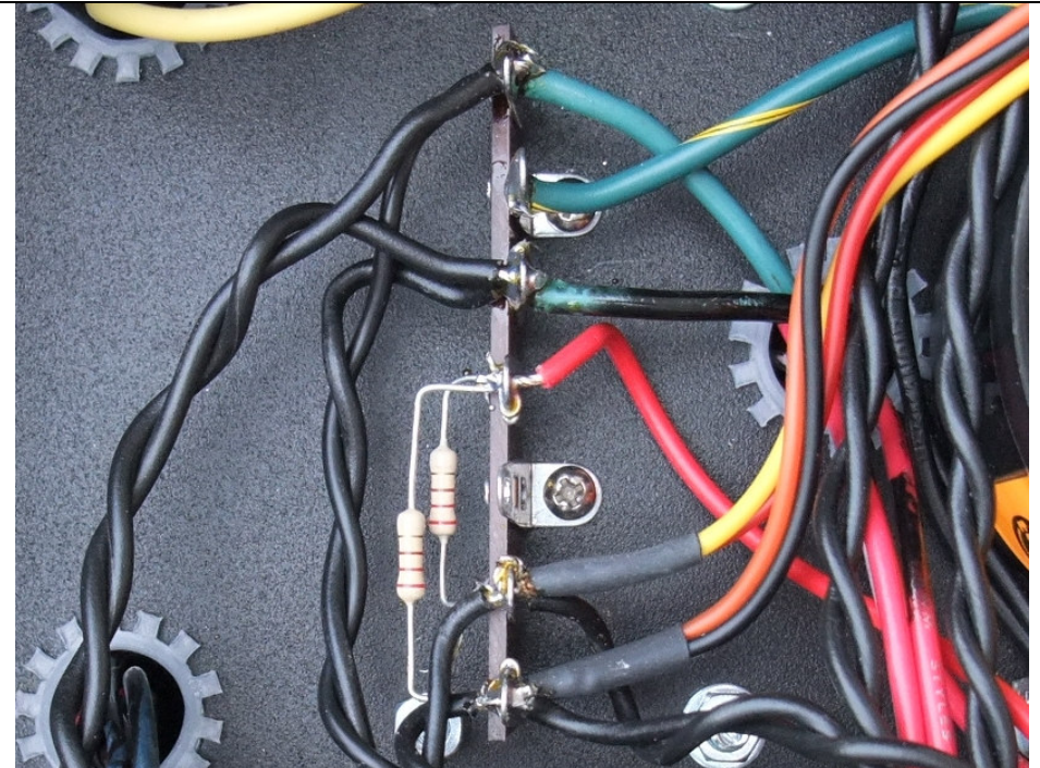
Barette relais 2 : raccordement des filaments
