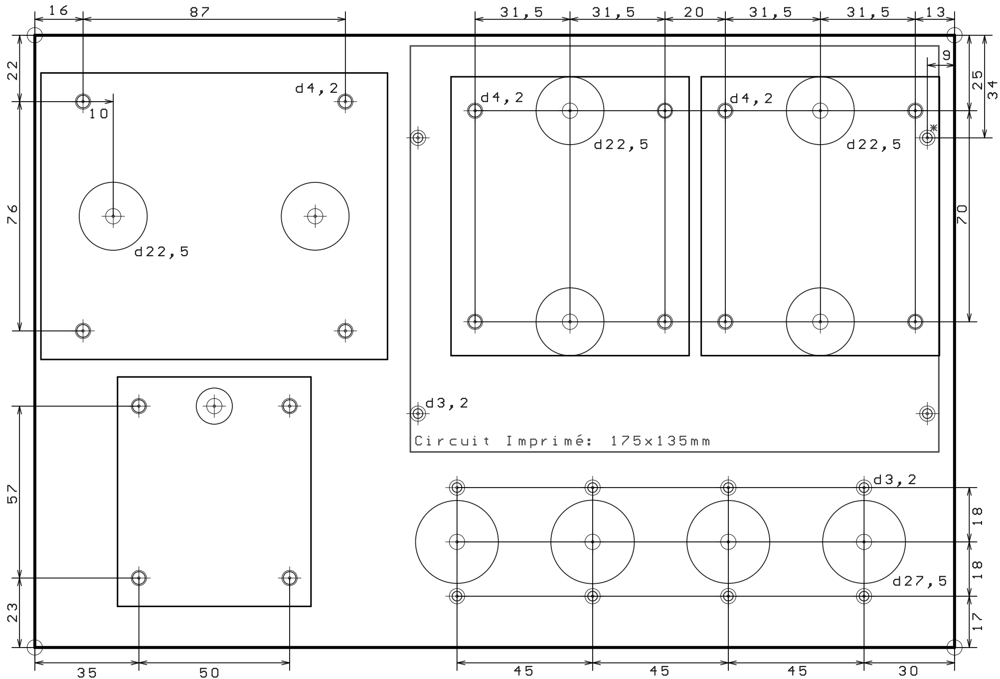
Dimensions mesurées à l'extérieur du châssis
